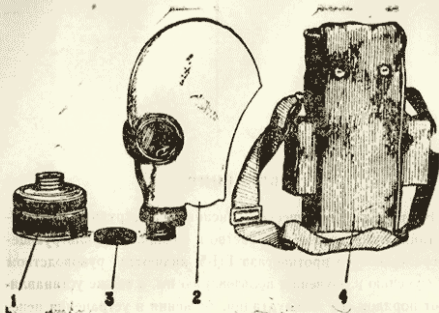
Рис. 1. Противогаз ГП-5:
